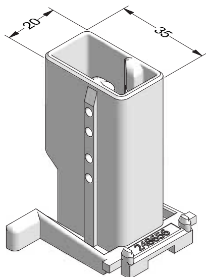
Механический соединитель импоста 78 РА
